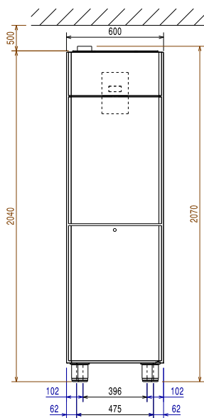
Alzado
